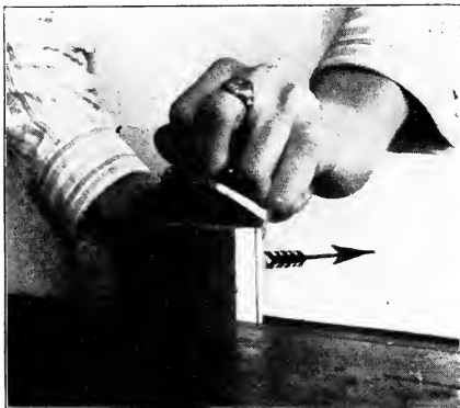
Fig. 83—Chamfering End
